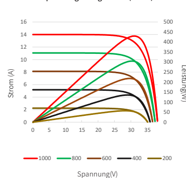
Strom-Spannungs- und Leistungs-Spannungs-Diagramme(430W)
